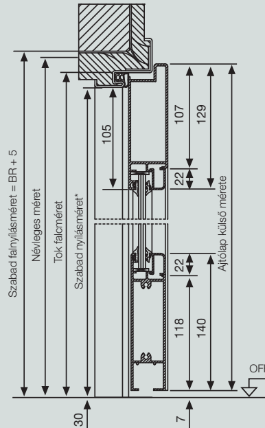
Kívánságra keresztbordával és felső ajtócsukóval (a füstgátló ajtóknál előírás).
