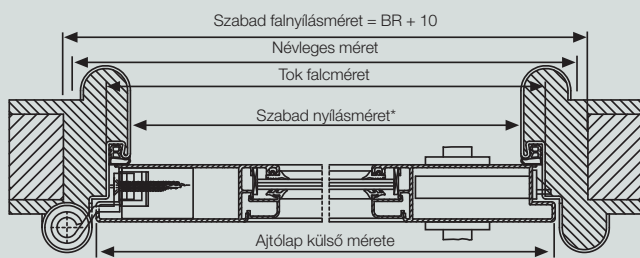
Roundstyle-tokkal és Glóbuszpánttal
